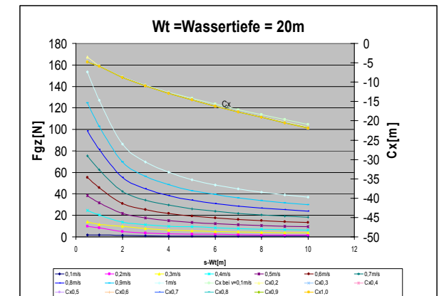
Berechneter seitlicher Versatz C_x [m] des Antennenkabels und erforderlicher Bojenauftrieb F_{gz} [N] bei Variation der Kabellänge s = Wt + 0,5m \dots + 10m und der Wassergeschwindigkeit v = 0,1 \dots 1m/s
