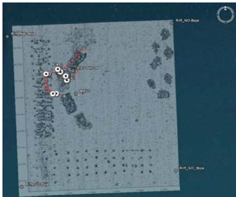
GPS-Track eines Tauchganges am künstlichen Ostseeriff Nienhagen Track und Foto-Wegpunkte überlagert ein Fächer-Echolothbild (Darstellung mit Hilfe von Google-Earth)
